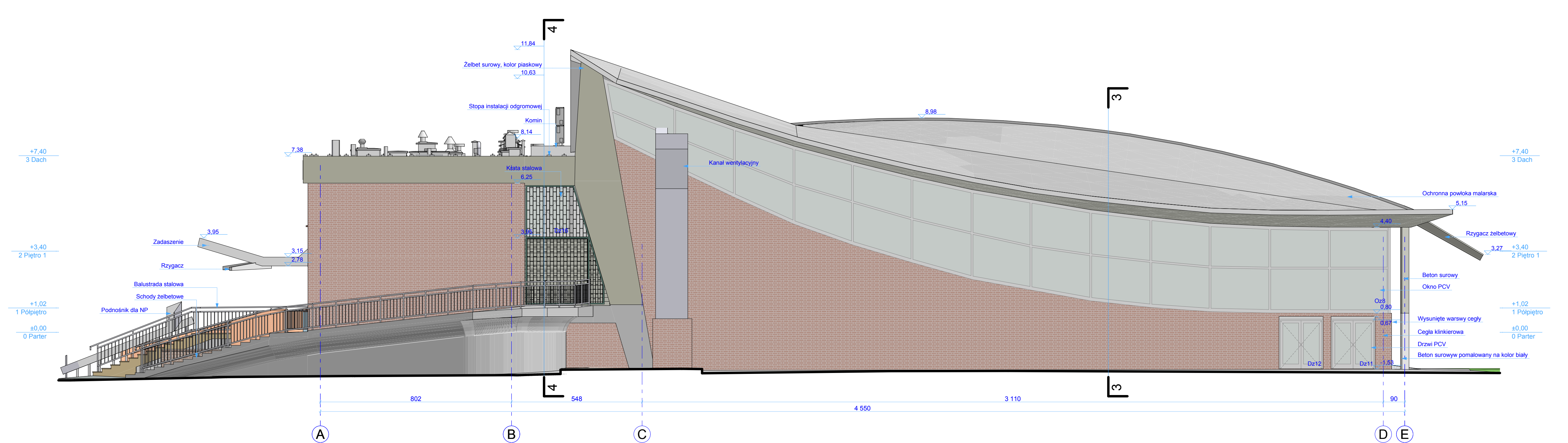
E-04 Elewacja południowo-zachodnia
